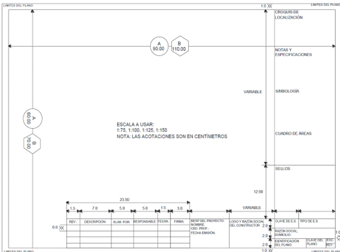
Características del plano del Proyecto arquitectónico.
