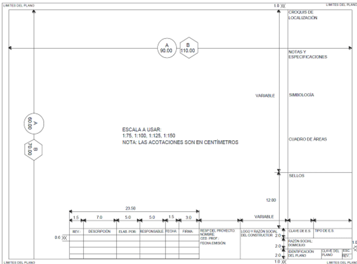
Características del plano del Proyecto arquitectónico.
