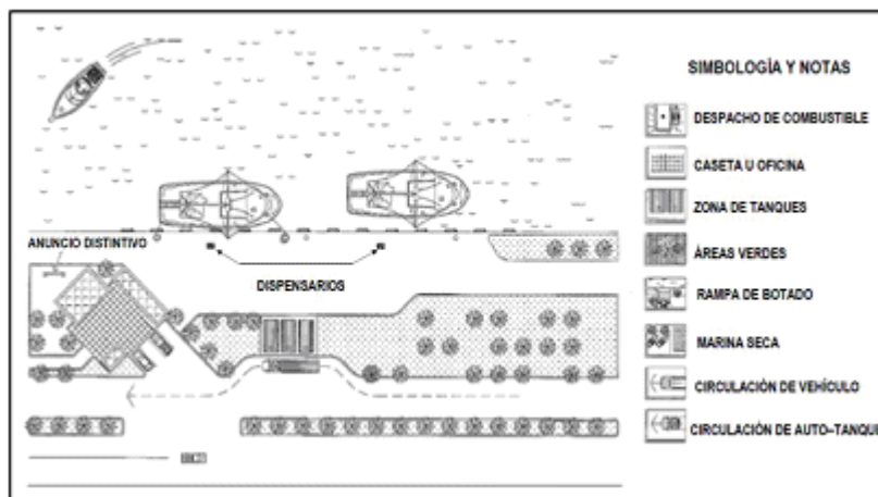
Figura 1. Disposición y arreglo típico para un muelle fijo marginal.
